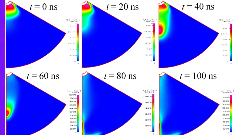
ストリーマ進展時の電子数密度分布の時間変化(数値解析)
