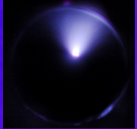
水蒸気中に生成したプラズマ
