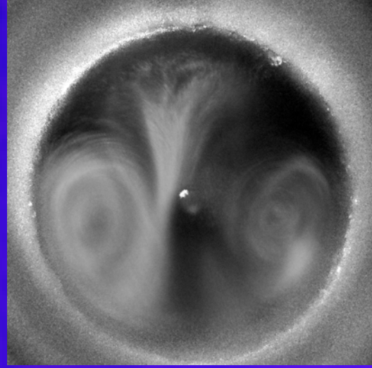
流動場: 双子渦の形成
