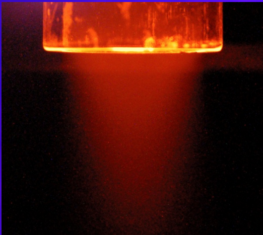
大気圧低温プラズマ流の可視化
