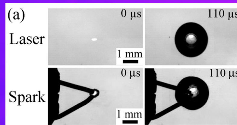
水中に形成される気泡の挙動
