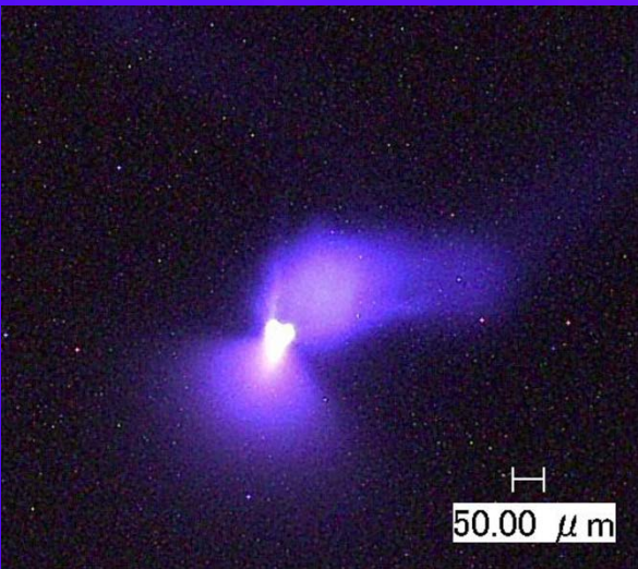
水蒸気中に生成したプラズマ
