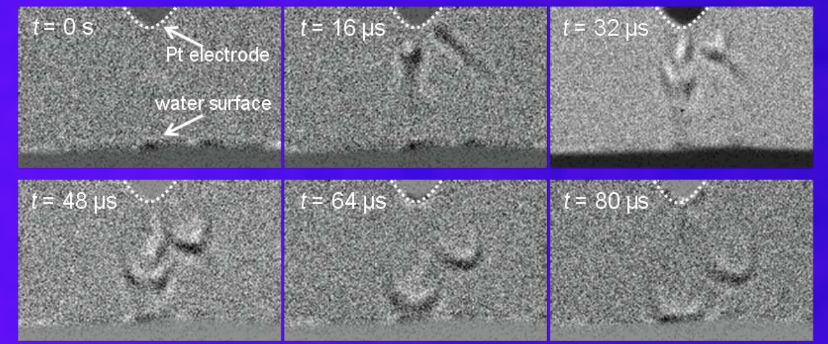
水面上のプラズマにより形成される熱流動場。秒速15 m/s程度の気流が放電時に発生する様子
