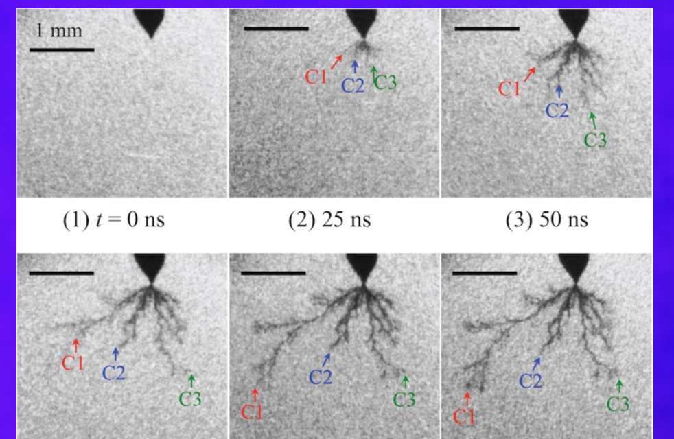
水中に形成される2次ストリーマ進展の様子
