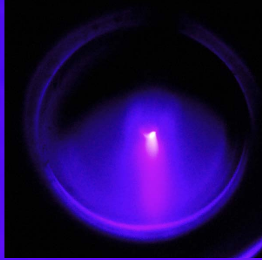
発光分布: 400nm
