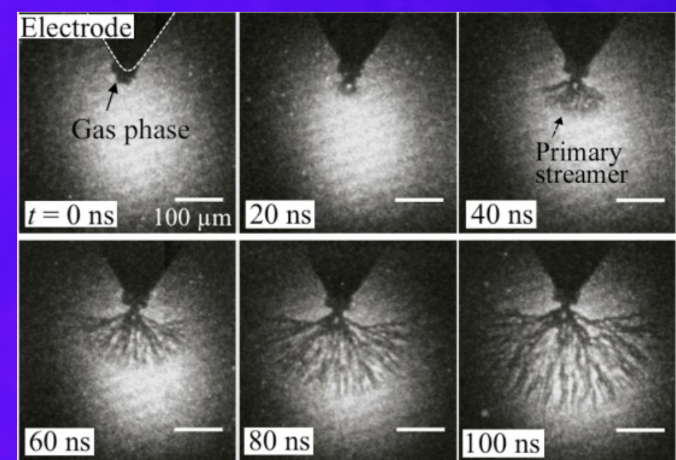
水中に形成される1次ストリーマ進展の様子
