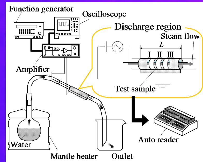
管内の水蒸気をプラズマ化し、滅菌を行う装置。
