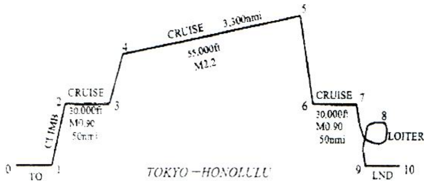
第2 図 飛行プロフィール
