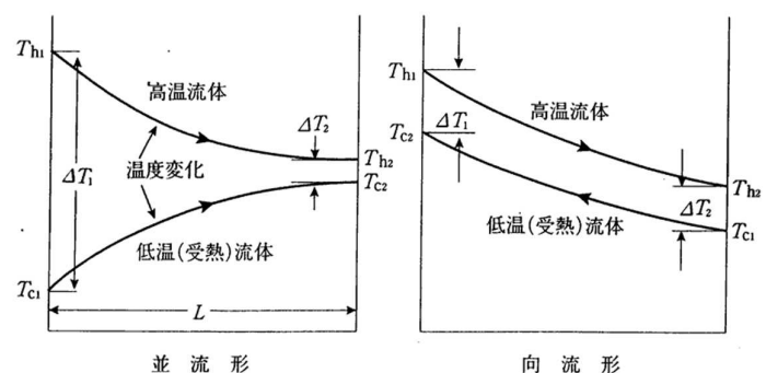
熱交換器内の温度変化
