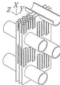
プレートフィンアンドチューブ型熱交換器
