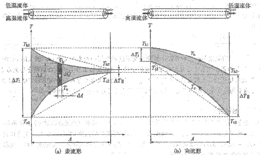
二重管式熱交換器の温度分布
