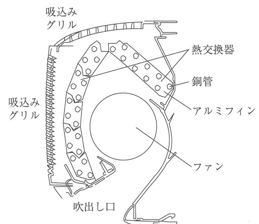
ルームエアコン室内機断面と熱交換器
