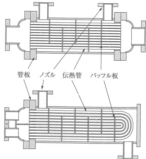
シェルアンドチューブ型熱交換器
