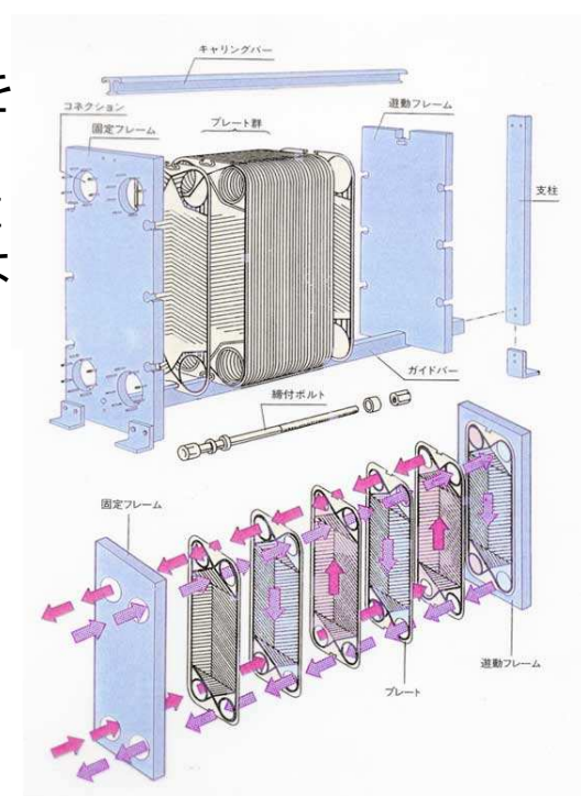
プレート式熱交換器の構造
