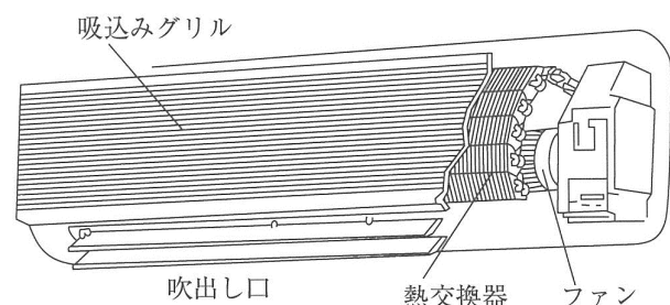
ルームエアコン室内機
