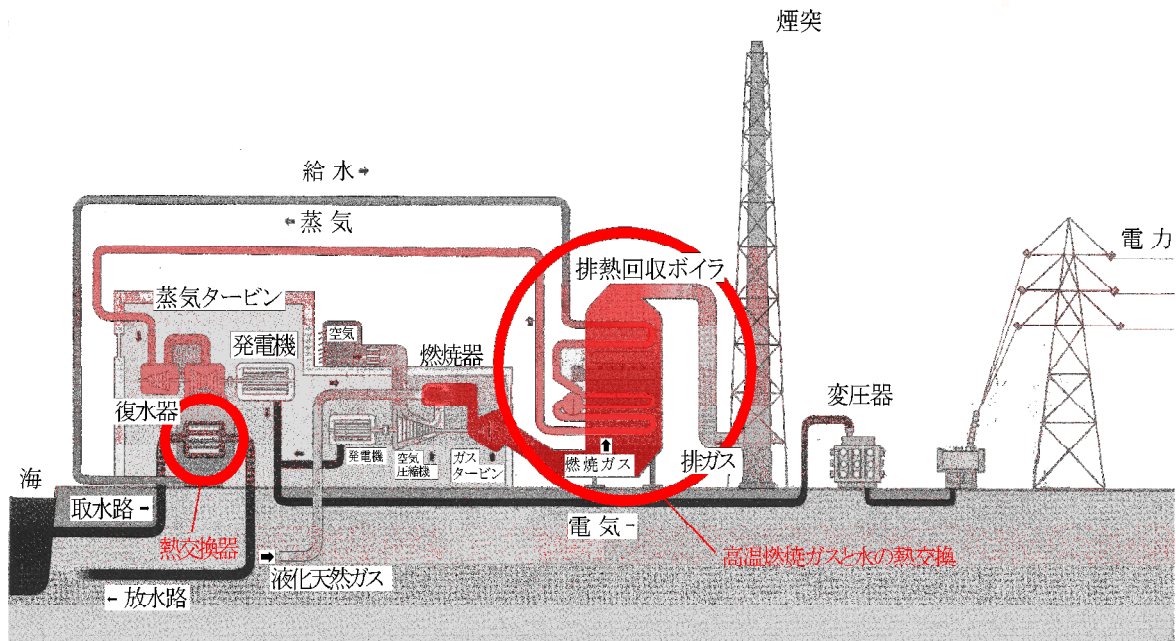
複合サイクルの熱交換
