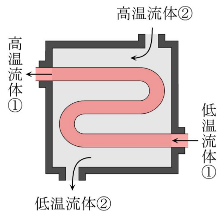
熱交換器の模式図
