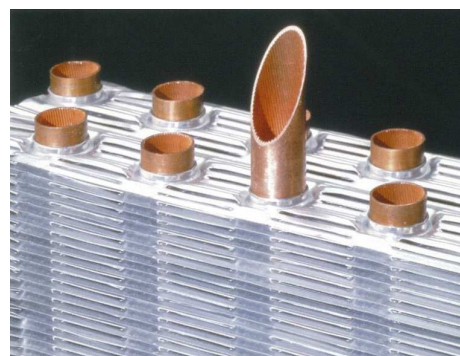
コンパクト熱交換器
