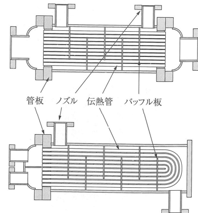
シェルアンドチューブ型熱交換器
