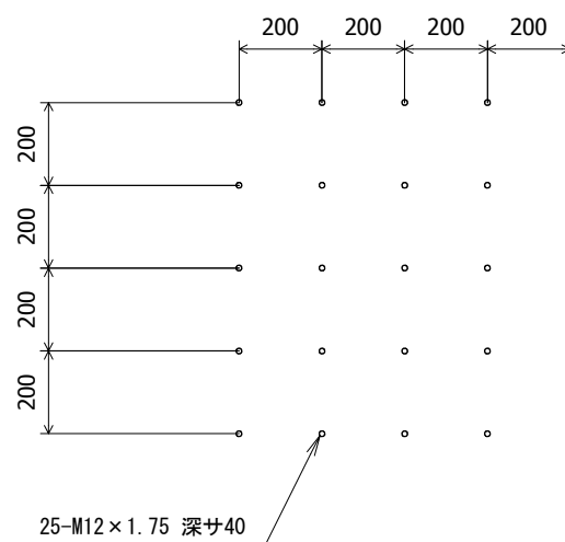
D-D ( 1 : 20 )
